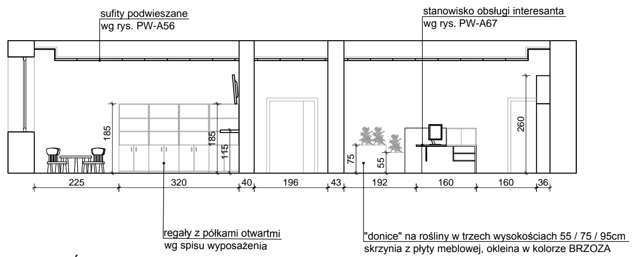
PRZEKRÓJ B-B
