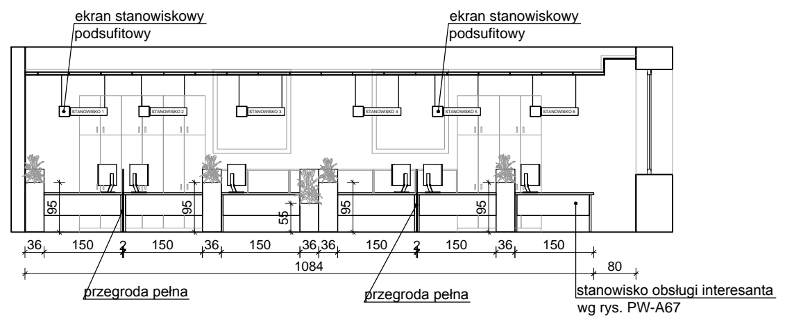
PRZEKRÓJ A-A
